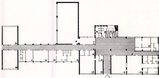
Földszinti alaprajz 1:800
