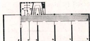
II. emeleti alaprajz 1:800
